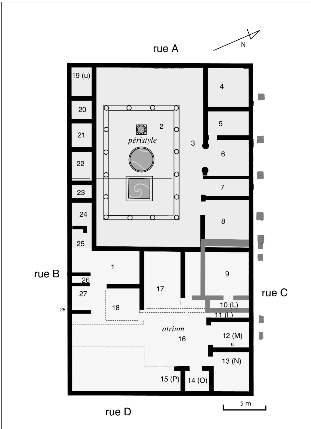
Fig. 9. Plan de la maison à Portiques du Clos de la Lombarde.
